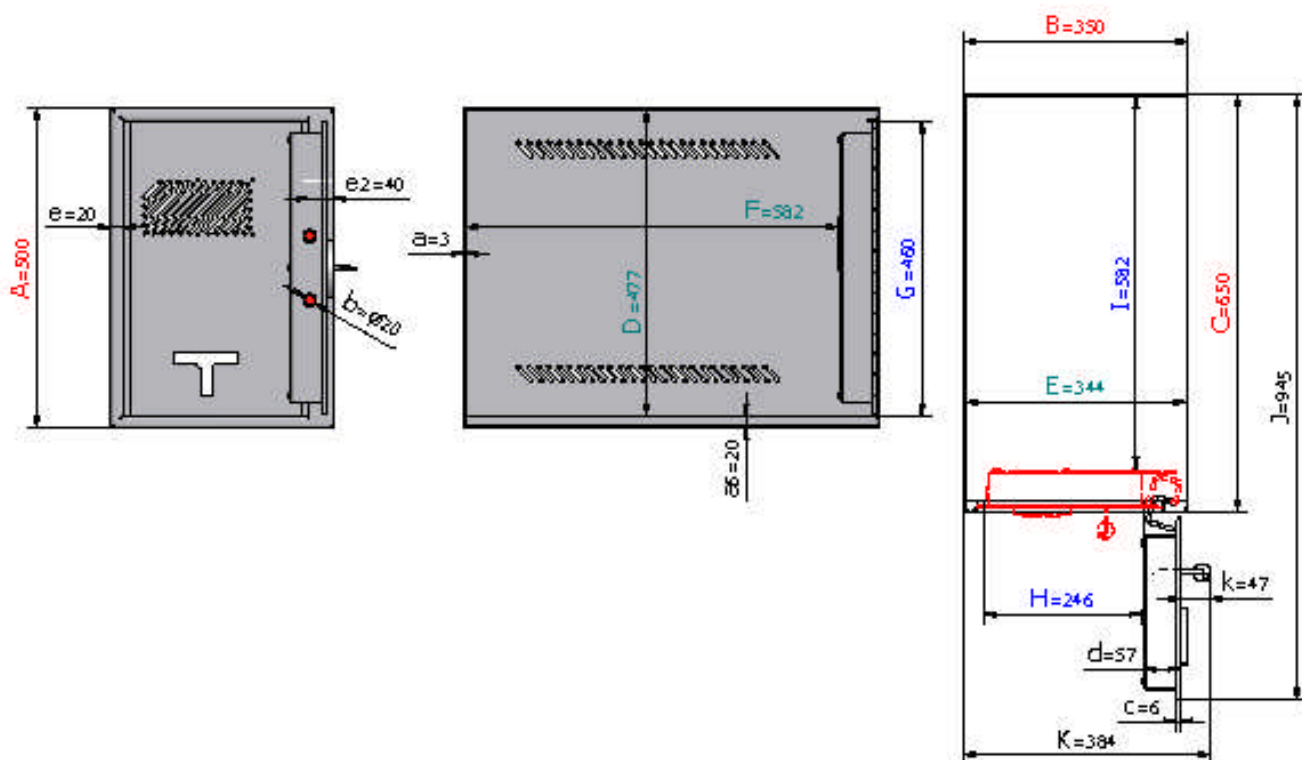
Frontansicht
